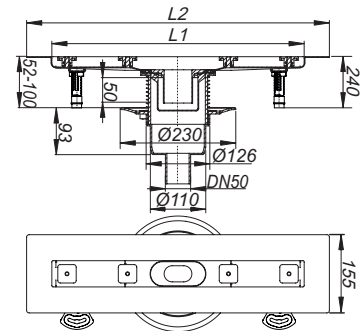
douchegoot CeraLine verticaal F 500 – 1200
