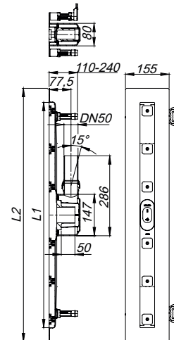
douchegoot CeraLine F 500 – 1200
