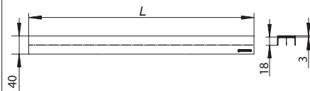
afdekplaat CeraLine mat zwart
