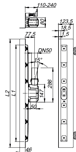
douchegoot CeraLine W 500 – 1200
